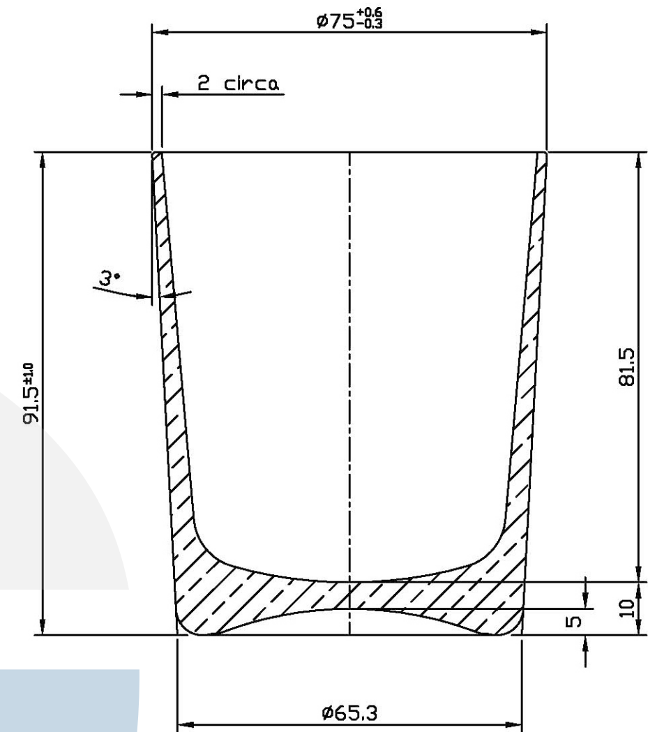
SEZIONE
